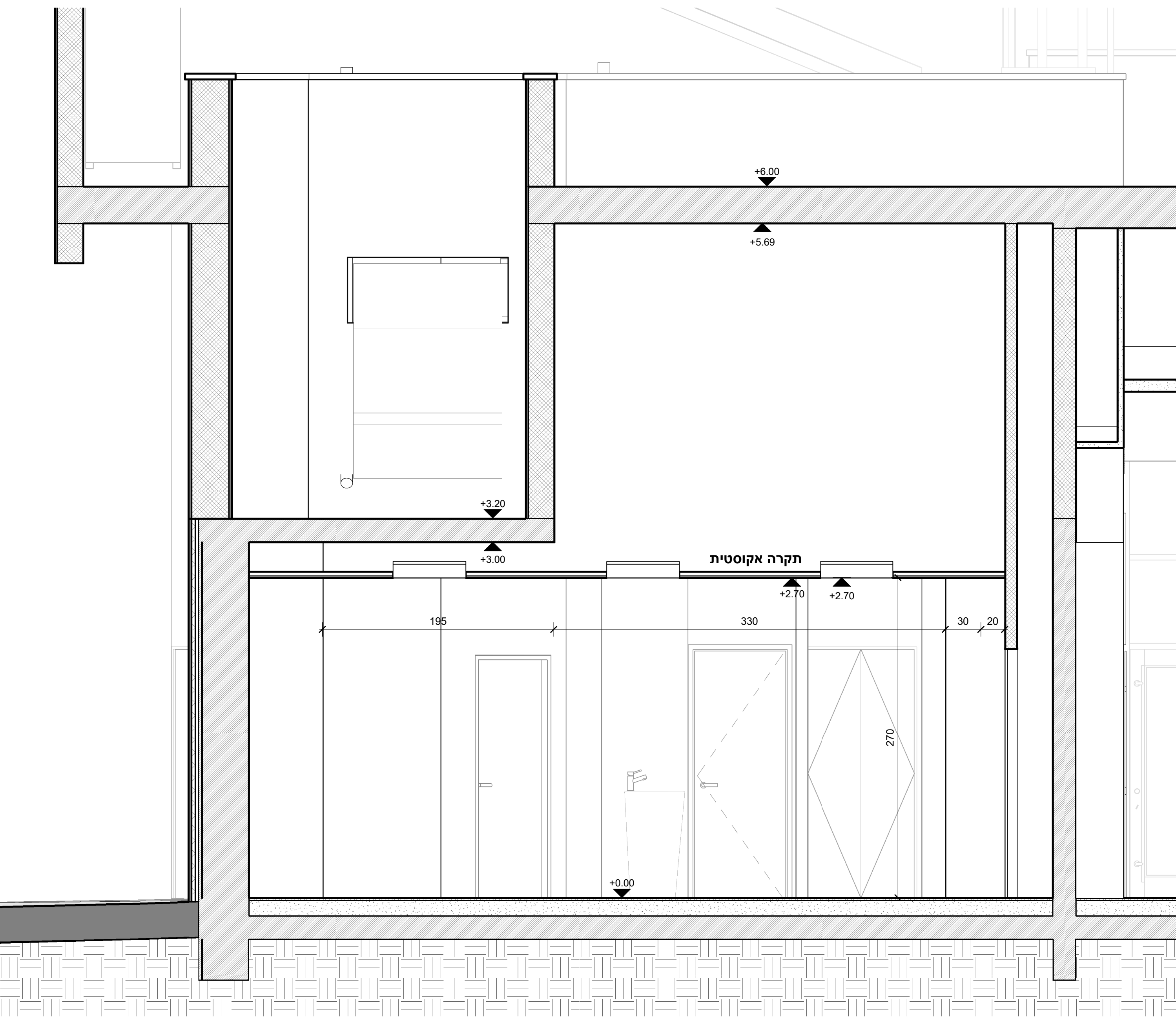
11-11 חתך ② 1 : 25
